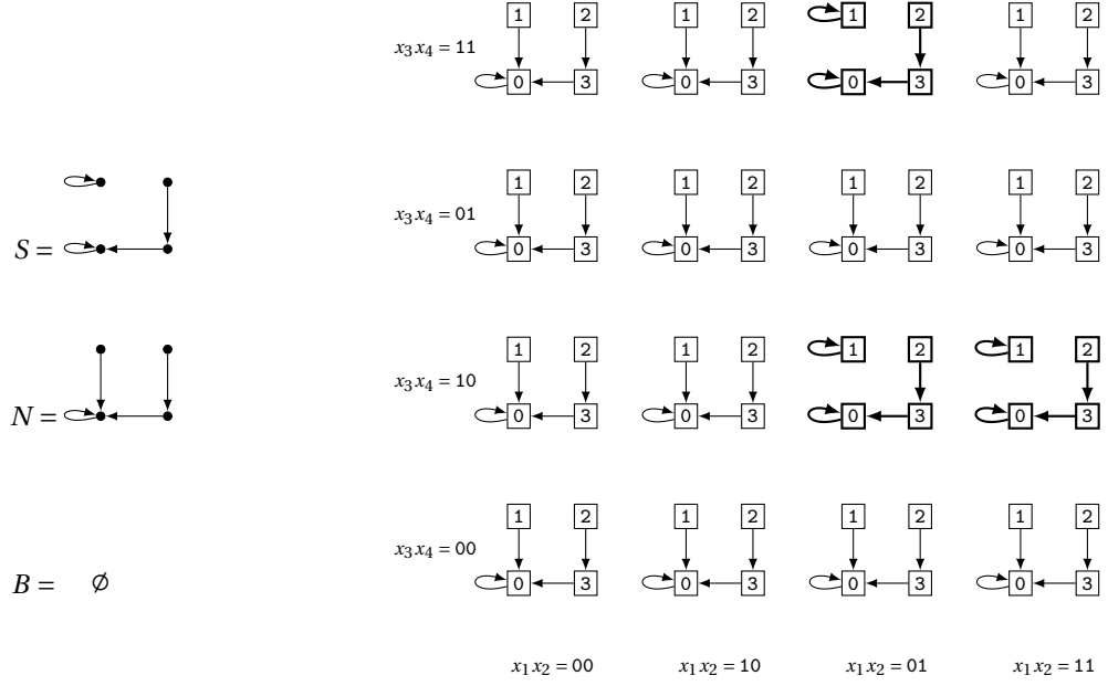
FIGURE 6.1. – Illustration de la construction du lemme 6.2, pour la propriété
