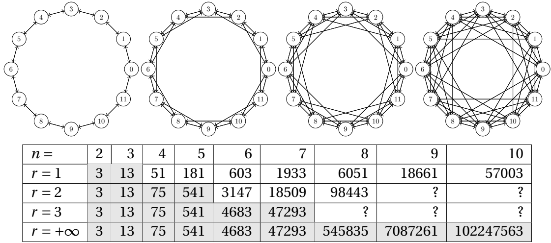
FIGURE 8.9. – Graphe d’interaction (sans boucle) pour les automates cellulaires élémentaires finis périodiques de rayon r = 1, 2, 3, 4 et n = 12 automates, et quelques comptages de \#GBS(G) réalisés par force brute. Pour n \leq 2r + 1 on obtient le graphe complet (cases grisées). On remarque que le nombre d’étiquetages \{\boxplus, \boxminus\} grossit beaucoup trop vite pour mon algorithme qui teste naïvement l’ensemble des sous-ensemble d’arcs (script python3 utilisant le package multiprocessing, sans élimination des symétries, lancé sur une machine à 40 processeurs; comptage pour rayon 2 à 8 sommets réalisé en environ 2 heures).
