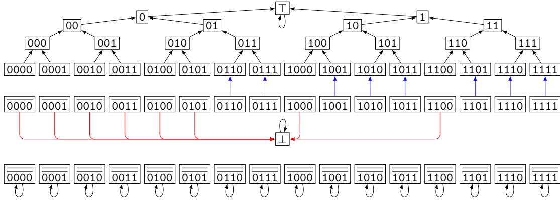
FIGURE 6.2. – Illustration de la construction du théorème 6.10, pour la formule :
