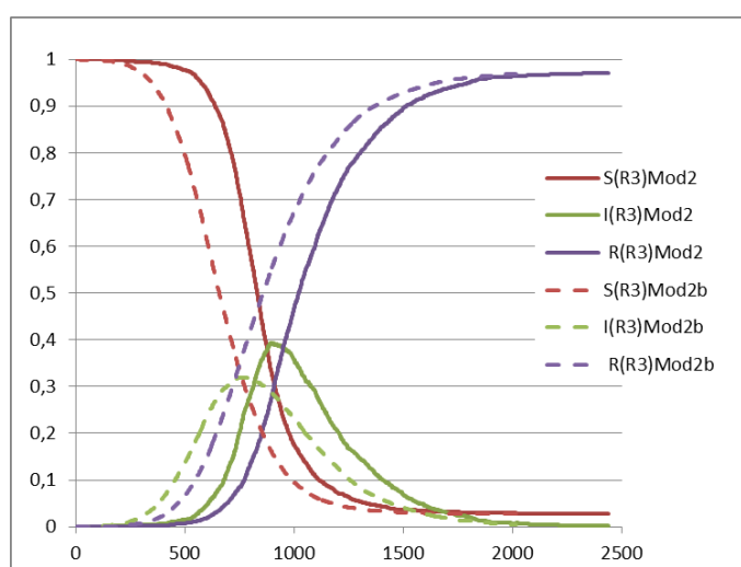
Figure 10. Comparaison de la version 2 et de la version 2bis du modèle distribué
