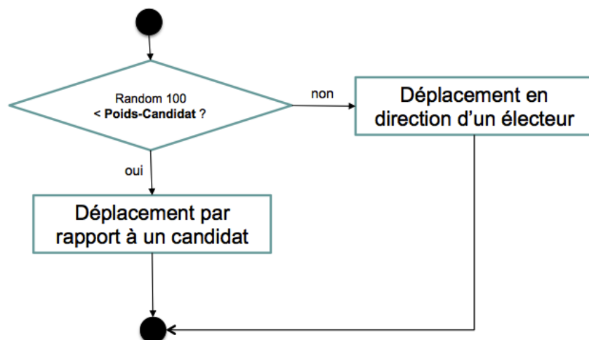
Figure 21. Description de la dynamique des électeurs
