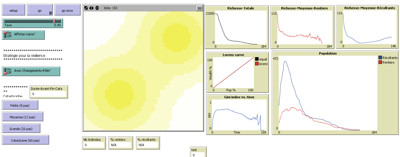
Figure 46. Le système s'effondre à 0.40
