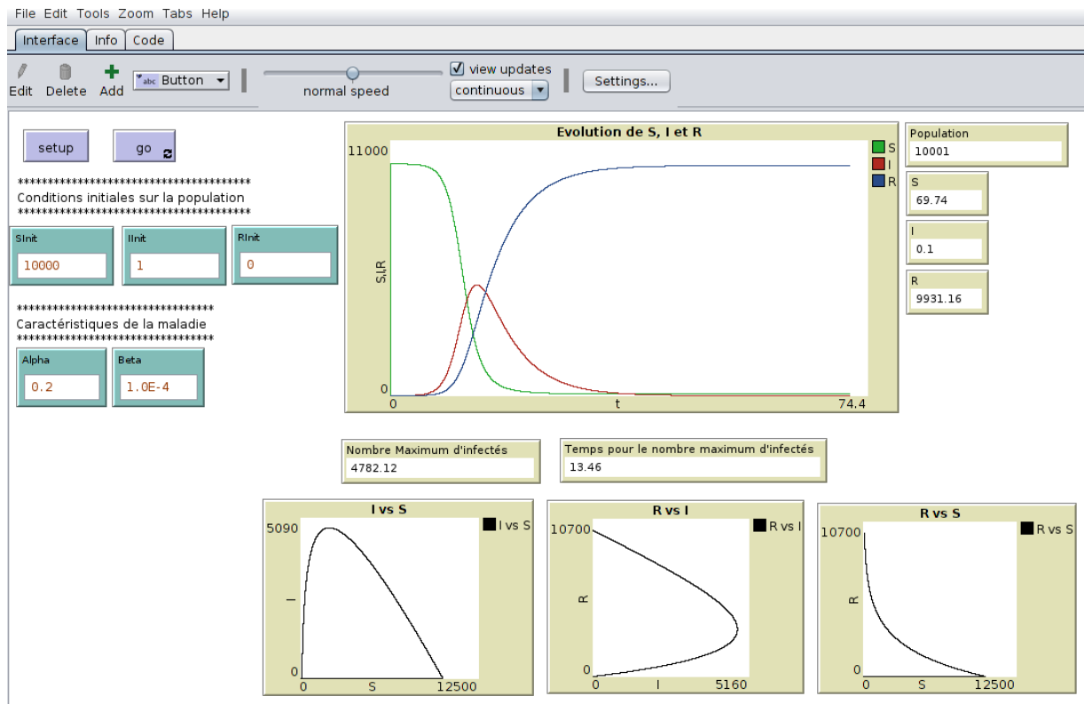
Figure 27. Capture d'écran de trajectoires obtenues par la méthode numérique de RK4 appliquée au modèle SIR. Ici, \alpha = 0.2 , \beta = 0.0001 , S_{init} = 10000 , I_{init} = 1 , R_{init} = 0
