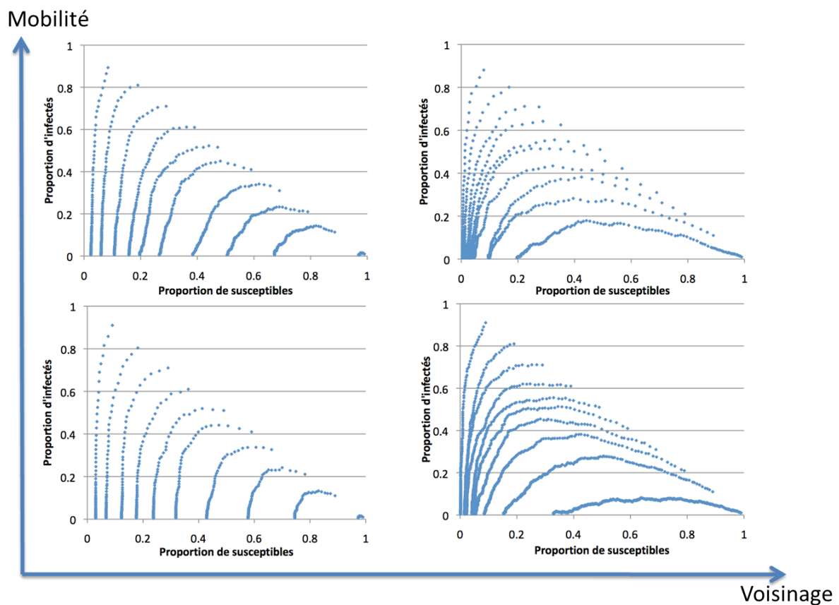
Figure 11. Conséquences de la mobilité et de l'augmentation du rayon de voisinage sur les trajectoires prises par le système
