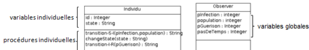
Figure 8. Diagramme de classes du modèle multi-agents
