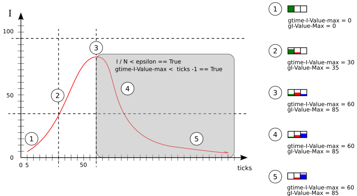
Figure 29. Illustration de la condition d'arrêt
