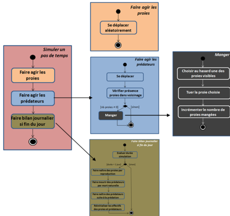
Figure 41. Détails des processus généraux du modèle micro .
