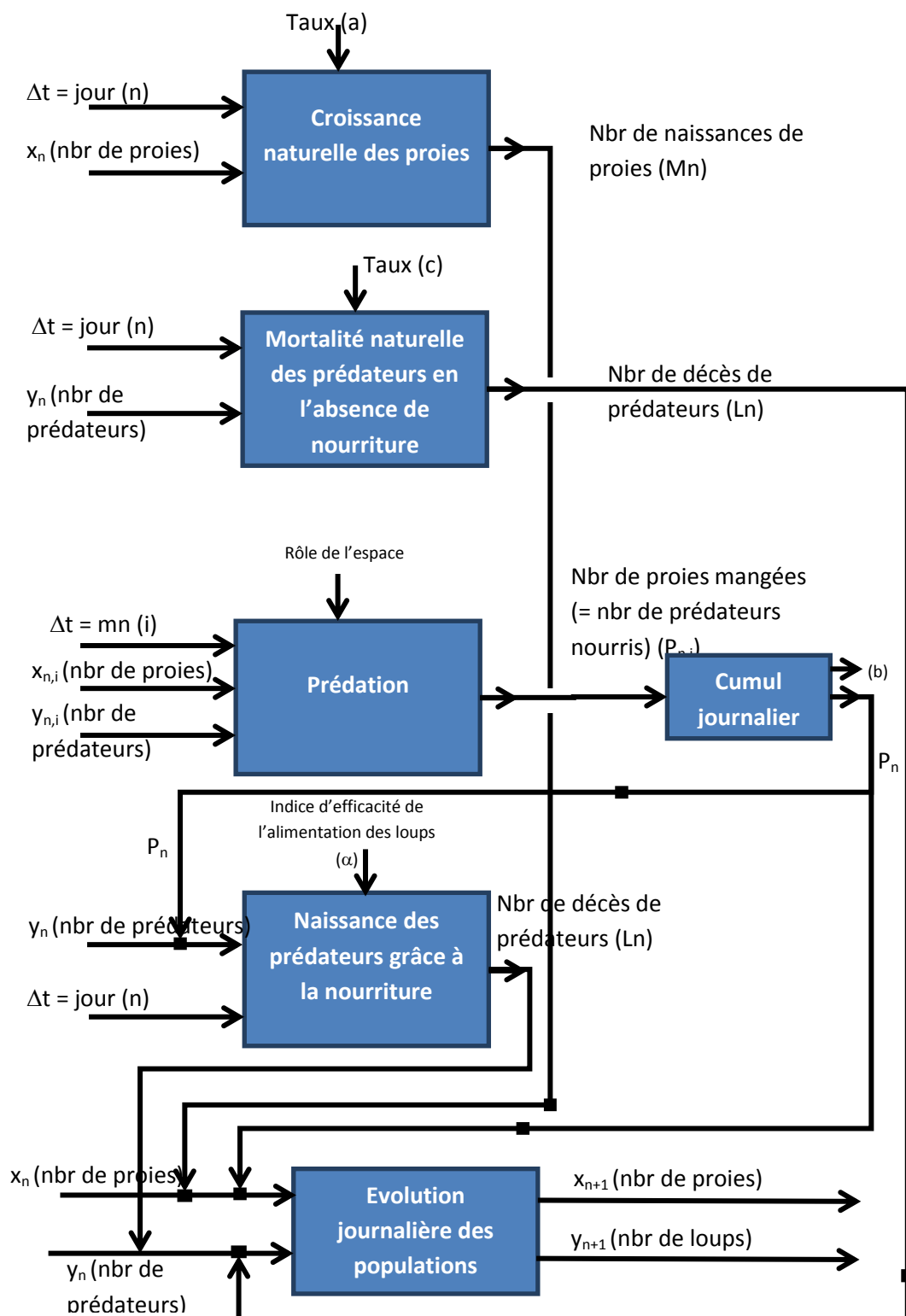
Figure 38. Diagramme d'activité (SADT) global du modèle proies-prédateurs
