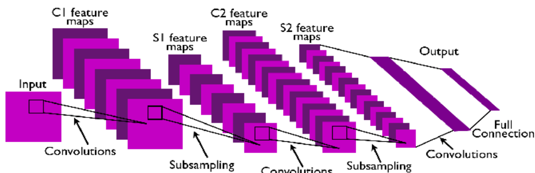
Illustration de l'alternance entre convolutions et normalisation / sous-échantillonnage amenant de l'image (input) à la classification (output). Image : Lecun, Yann, Koray Kavukcuoglu, Clement Farabet, « Convolutional Networks and Applications in Vision », op. cit.
